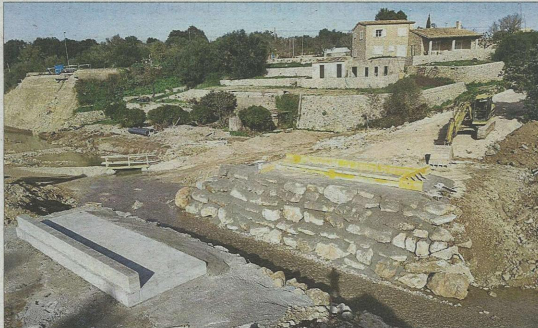
Los trabajos previos dejan a punto la zona para la colocación del puente. CONSELL
